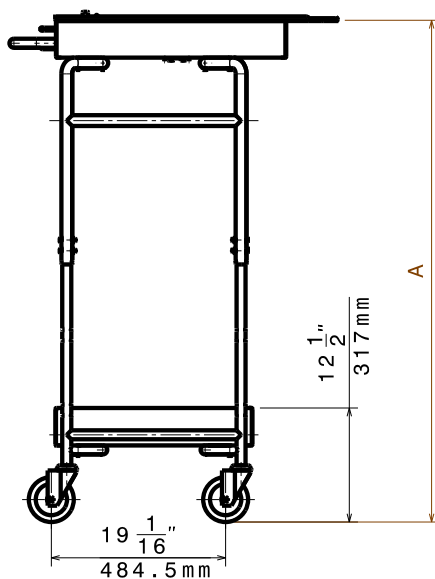
Zij aanzicht
